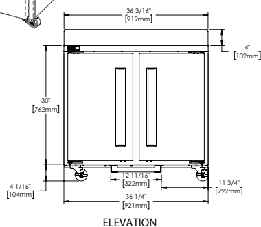
ELEVATION
