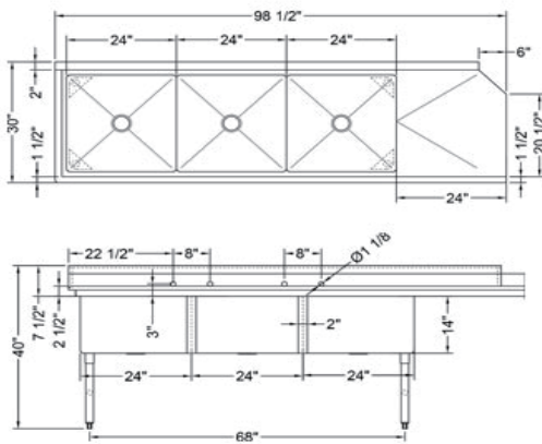
SI824-3L-DW DIMENSIONS
