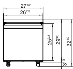
AUF27SD
