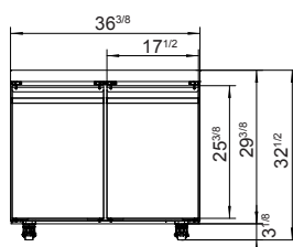
AUF36SD
