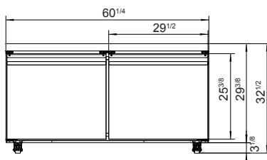
AUF60SD
