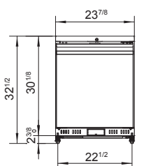
AUF24SD
